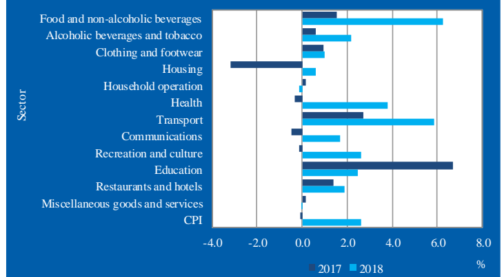
Figure 4: \Delta I per sector for April, 2017- 2018
